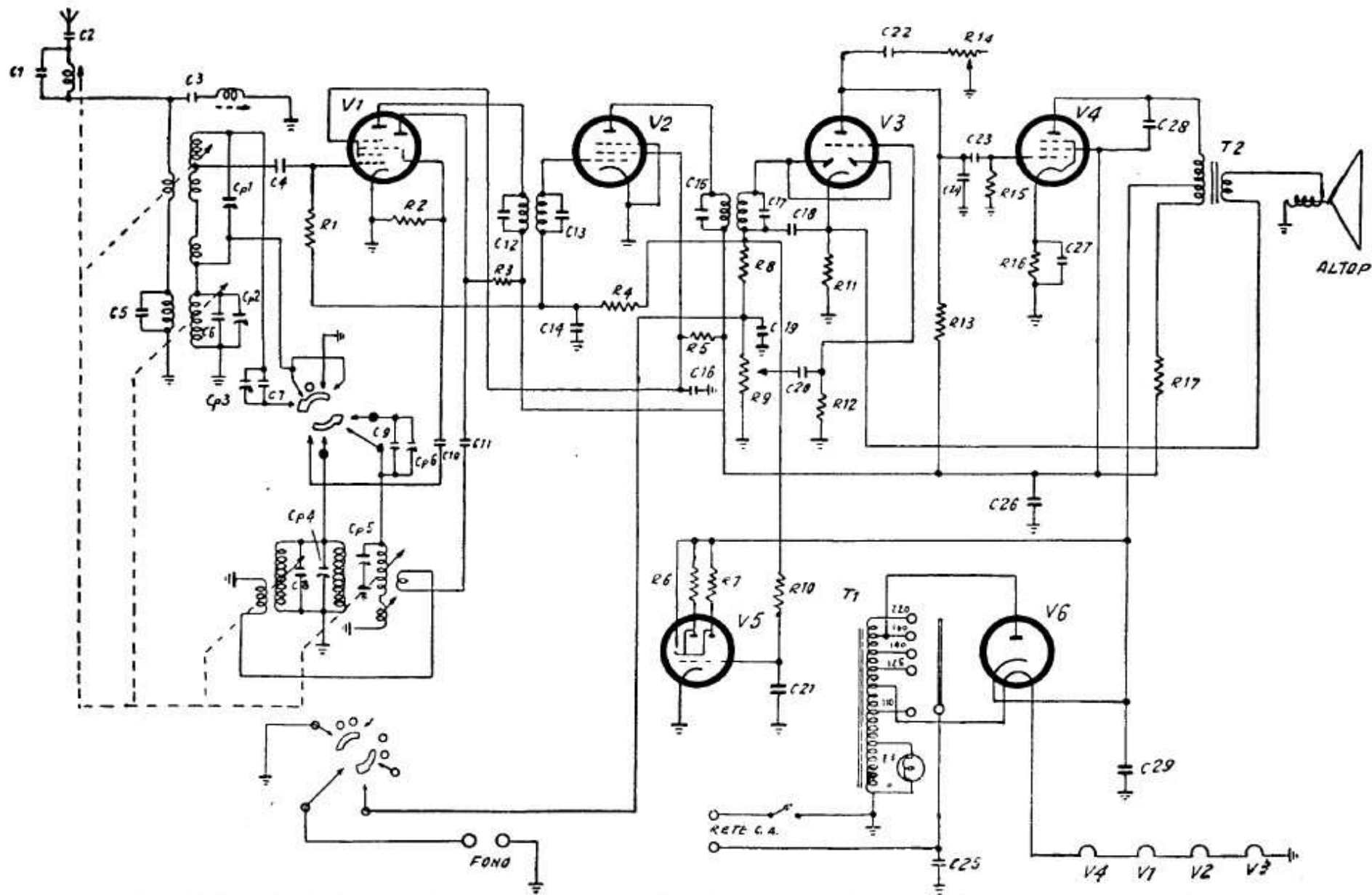
ALLOCCIO BACCHINI - Mod. 426. Una gamma onde medie e due gamme onde corte. Media frequenza 465 kc/s. (Vedi a pag. 20 tabelle valori e taratura).
